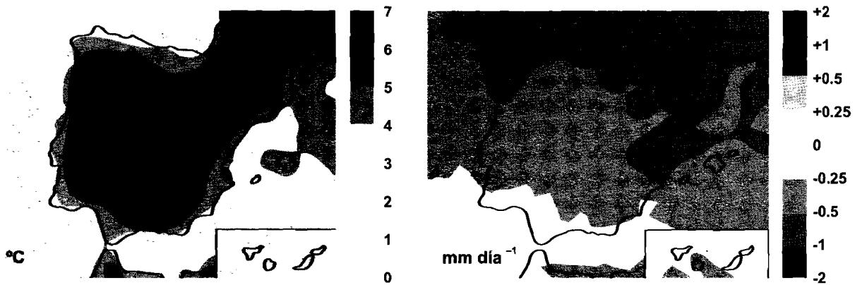
Figura 1. Escenarios de temperatura y precipitación en España para el último tercio del siglo XXI. Simulaciones realizadas bajo un escenario de emisiones elevadas de CO 2 (escenario A2) a partir del período de referencia 1961-1990 por el Grupo de Modelización Numérica para el Medio Ambiente y el Clima, UCLM, Toledo (Castro et al. 2004)
