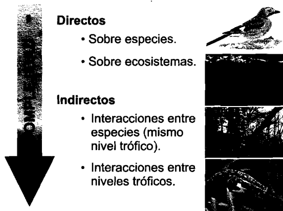
Figura 6. Los efectos del cambio global se vuelven más complejos y por tanto más difíciles de comprender y anticipar a medida que pasan de ser directos a indirectos o de afectar a una especie o a todo un sistema de especies que interaccionan entre sí. En realidad, el cambio global afecta a todo el sistema y tiene efectos tanto directos como indirectos, pero por razones prácticas con frecuencia resulta operativo trabajar a distintos niveles de complejidad y realismo.
